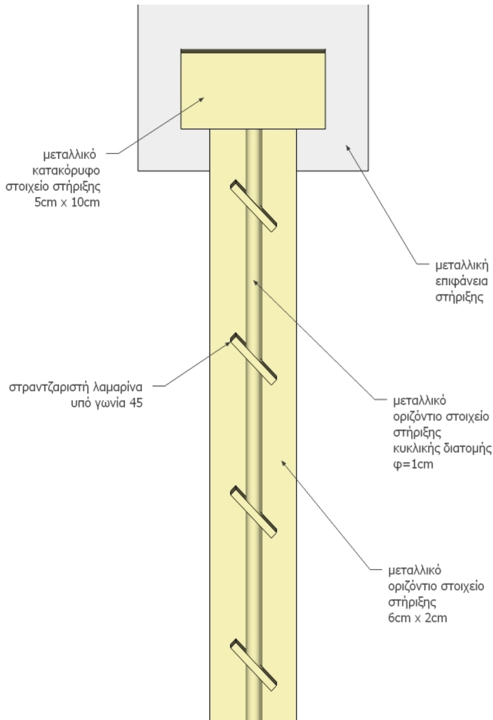
ΕΙΚΟΝΑ 4. ΛΕΠΤΟΜΕΡΕΙΑ PANEL. ΚΑΤΟΨΗ.
